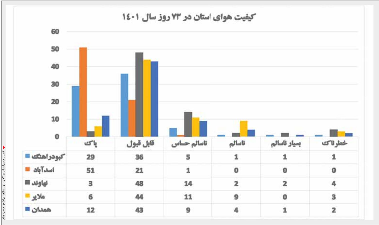
کیفیت هوای استان در ۲۳ روز سالخیز استان همدان
